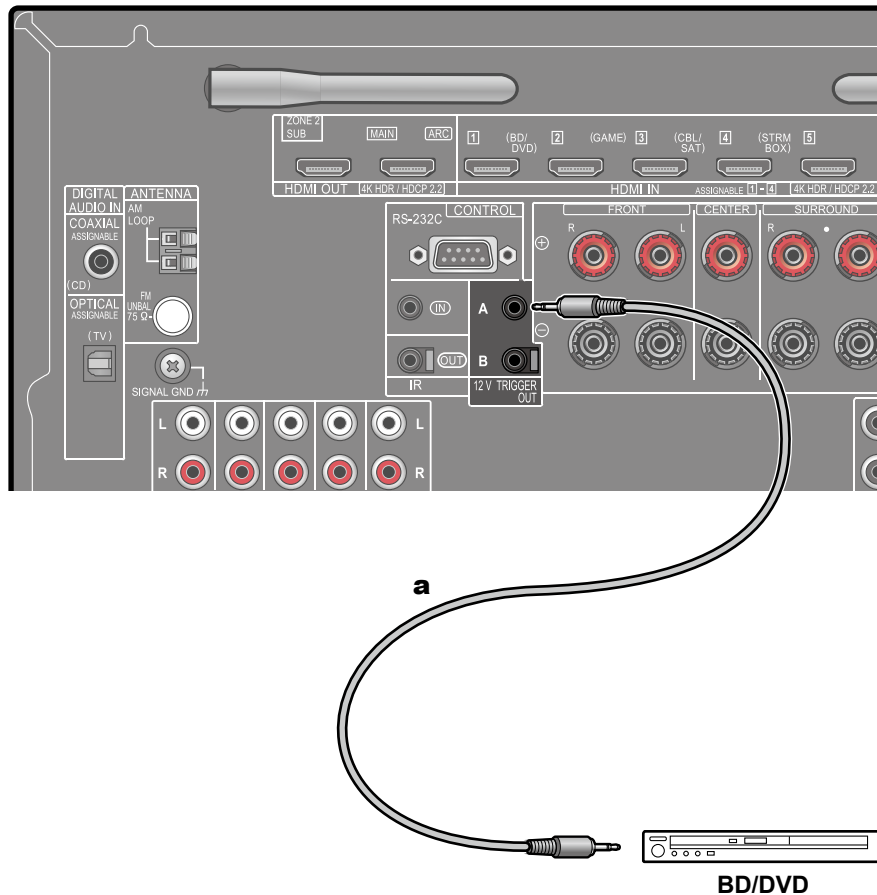
a Câble mini-prise monophonique ( \varnothing 1/8''/3,5 mm)
